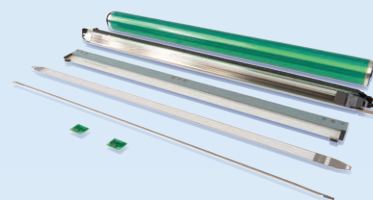
ZESPOŁY BĘBNA
